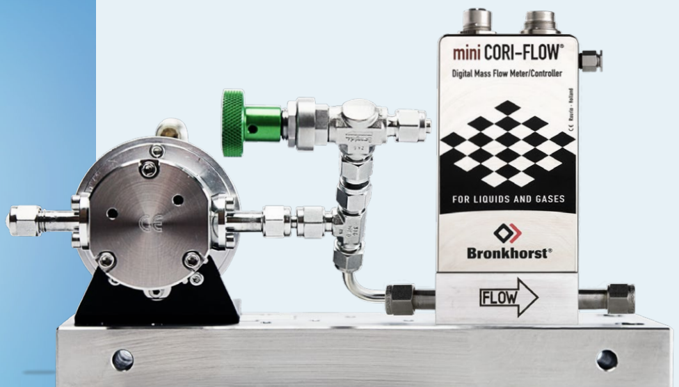
科里奥利流量计与定量给料泵组合
